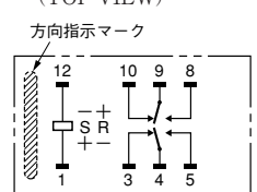
端子配置/内部接続図 (TOP VIEW)
