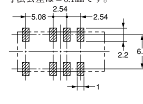
プリント基板加工寸法(TOP VIEW) 寸法公差は±0.1mmです。
